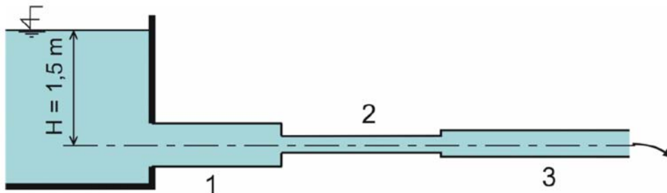
Slika 2: Skica vodovodnega omrežja
