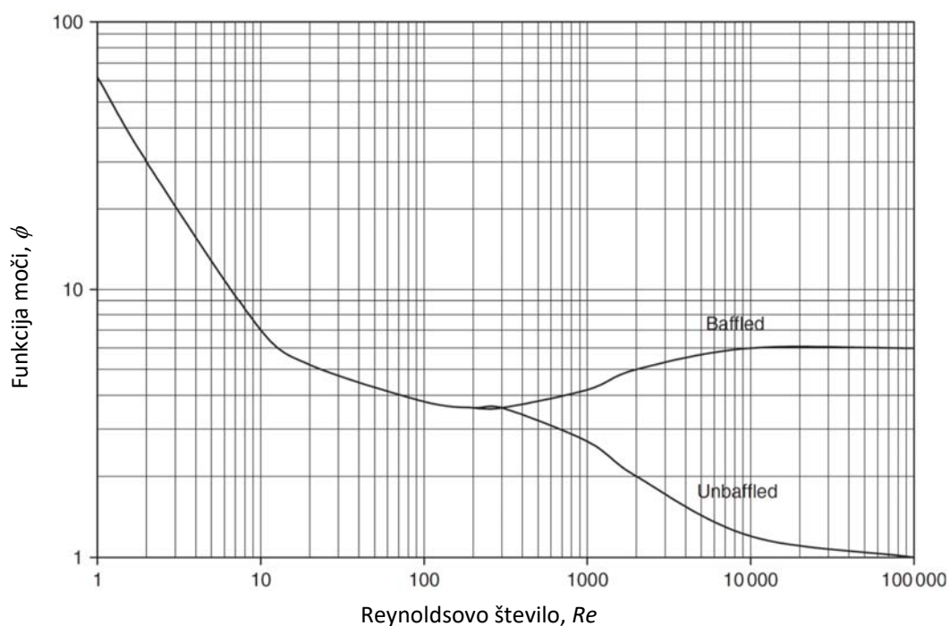
Slika 4: Graf funkcije moči za turbine v reaktorju s pregradami (baffled) in brez pregrad (unbaffled).
