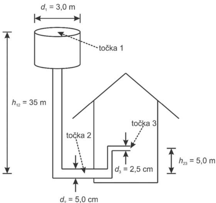
Slika 1: Skica poti vode od zalogovnika do pipe.
