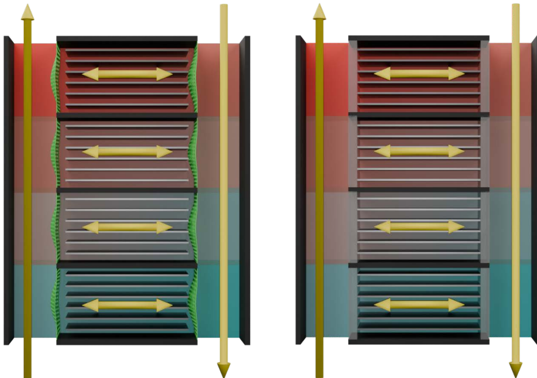
Slika 4: Prerez dveh različnih Hyperegov: v kratkih ločenih segmentih tekočina oscilira vzdolž trdninskih ploščic s pomočjo poroznih membran (levo) ali batov (desno). Prečno pa sta vzpostavljena dodatna tokova, ki oblivata posamezne segmente in dodatno ustvarjata temperaturni profil tako, da je najnižja temperatura v spodnjem desnem delu Hypereg, najvišja pa v zgornjem levem.
