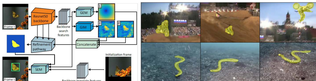
Slika 12: Arhitektura D3S (levo) in primeri lokalizacije objektov (desno).
