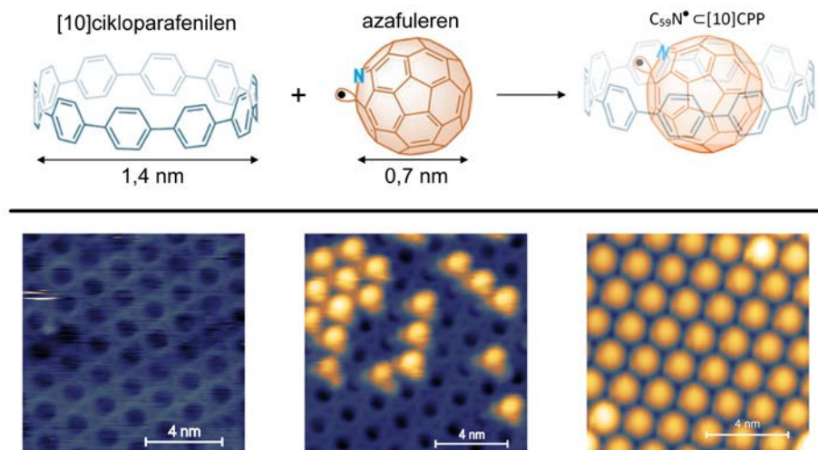
Slika 8: Kompleksacija azafulerena in [10]cikloparafenilena (zgoraj); populacija dvodimenzionalne mreže molekul [10]cikloparafenilena z azafulerenskimi radikali (spodaj)
