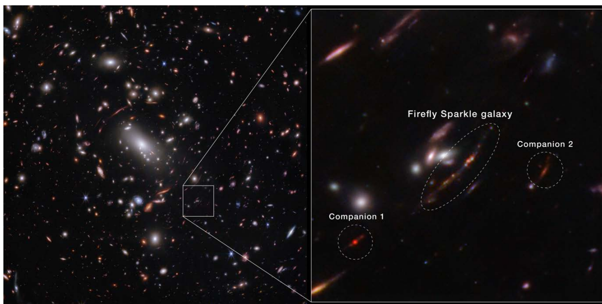
Slika 1: Na levi strani fotografije je jata galaksij MACS J1423, ki močno ukrivlja čas in prostor. Tako omogoča, da vidimo precej bolj oddaljene galaksije v ozadju. Ena izmed takih galaksij je Roj Kresničk (Firefly Sparkle galaxy) na desni strani. V njeni bližini sta še dve manjši galaksiji (Companion 1, Companion 2). Vir: NASA
