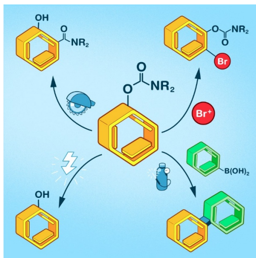
Slika 3: Stiliziran izbor pretvorb ArOAm funkcionalne skupine, kot jih vidi ilustrator Matej de Cecco.
