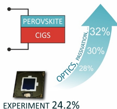
Slika 5: Izdelava rekordne, 24,2 % perovskitno-CIGS tandemske sončne celice ter optimizacija optike tandemske strukture za poti proti 30 % učinkovitosti pretvorbe. Avtor: dr. Marko Jošt
