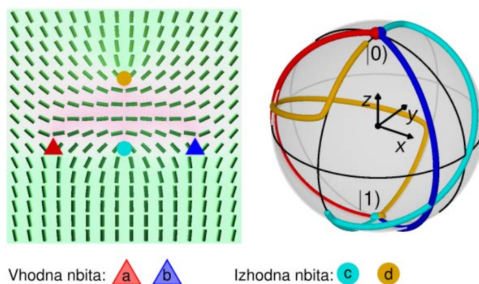
Slika 10: Izbrani defekti znotraj orientacijskega polja nematskega tekočega kristala služijo kot vhodni in izhodni nematski biti (nbiti) računske operacije. Enotska sfera kaže deformacijo, ki jo posamezni nematski biti opravijo med izvedbo logične operacije.
